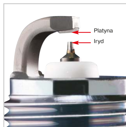
Elektroda środkowa ze stożkiem irydowym oraz elektroda masy z płytką platynową zapewniają najwyższą sprawność zapłonu w całym okresie eksploatacji świecy zapłonowej LPG LaserLine.
