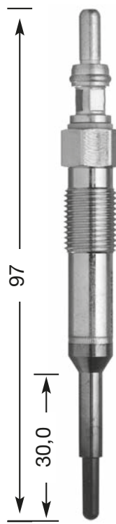
CZ 104 M 10 x 1.0 10 Hex 7 V
