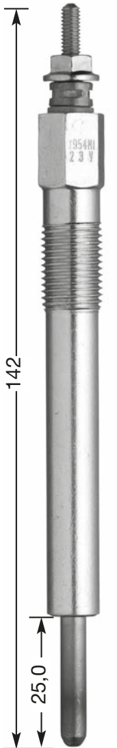
Y-954 M1 M 12 x 1.25 12 Hex 23 V
