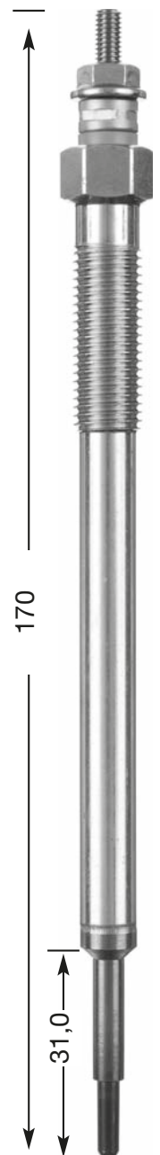
CZ 251 M 10 x 1.25 12 Hex 11 V
