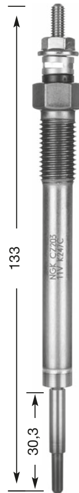
CZ 203 M 10 x 1.25 12 Hex 11 V
